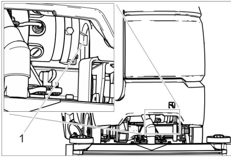
1 Важіль розблокування
